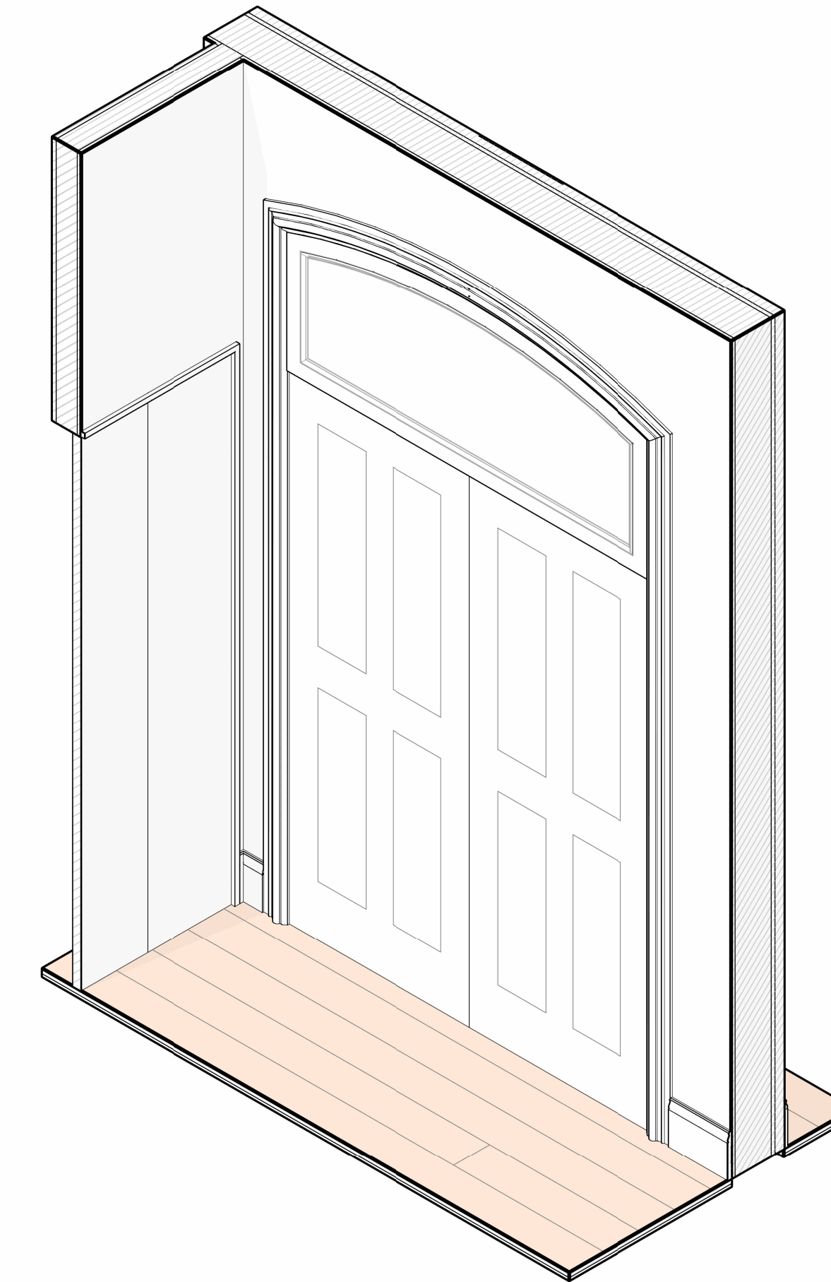
3 DOOR 13.1 - VESTIBULE SIDE AXON
